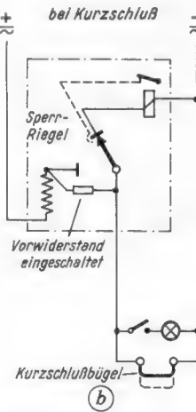
Bild 1b. Die gleiche Vorrichtung, jedoch im Falle eines Kurzschlusses. Das Relais ist ohne Strom; dieser setzt erst nach Beseitigung des Kurzschlusses ein
