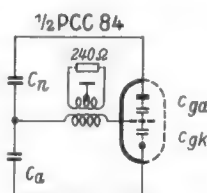
Bild 1. Neutralisierung der Gitteranodenkapazität der Katodenbasis-Stufe
