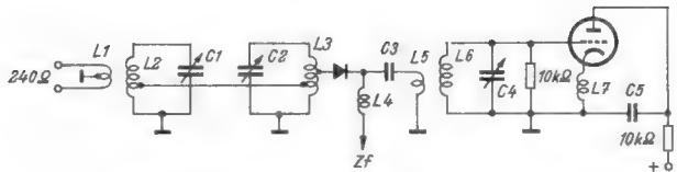
Bild 2. Prinzipschaltung des Abstimmteiles
