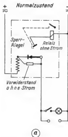
Bild 1a. Die automatische Sicherungseinrichtung im Normalzustand
