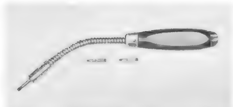
Bild 4. Schraubenzieher mit flexiblem Schaft und auswechselbaren Schneideneinsätzen von F. Damm, Remscheid
