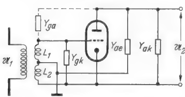
Bild 5. Zwischenbasisschaltung
