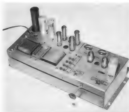
Bild 1. Musikbox-Verstärker von Klein & Hummel
