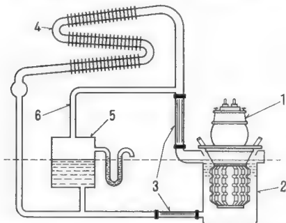
Bild 1. Der Wasserumlauf bei der Siedekühlung von Senderöhren hoher Leistung
