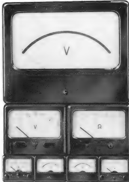
Bild 9. Beispiel für übersichtliche und raumsparende Anordnung rechteckiger Schalttafelinstrumente von Neuberger
