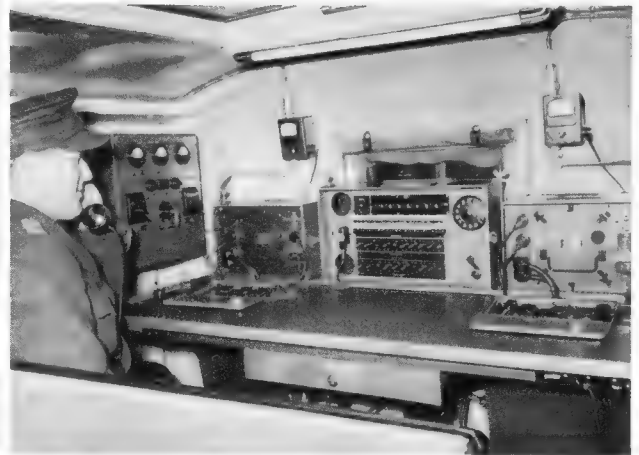
Links: Bild 7. 15-Watt-Funksprechgerät FuG 7 von Telefunken für transportablen Einsatz Rechts: Bild 8. Fahrbare Zentrale für ein Funknetz mit FuG 7
