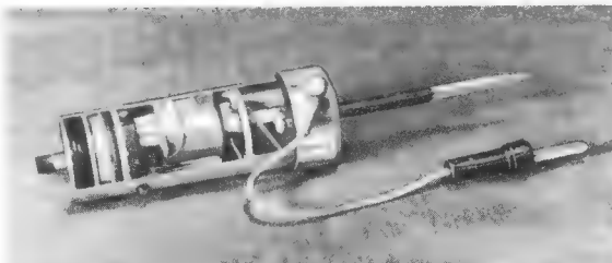
Links: Bild 6. Hochwertiger AM-Meßsender mit Schwebungssummer von Neuwirth
