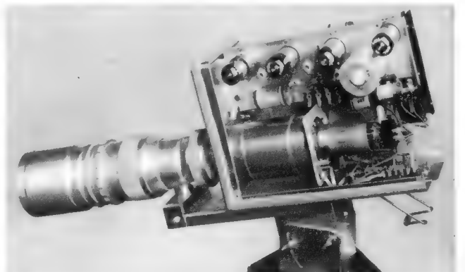
Bild 10. Blick in die Tekade-Fernsehkamera für industrielle Zwecke mit aufgesetztem Tele-Objektiv 135 mm
