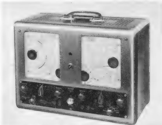
Links: Bild 4. Elektronischer Schalter von Siemens für Elektronenstrahl-Oszillografen
