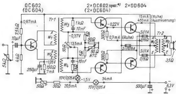
Bild 5. 4-Watt-Verstärker mit Telefunken-Transistoren
