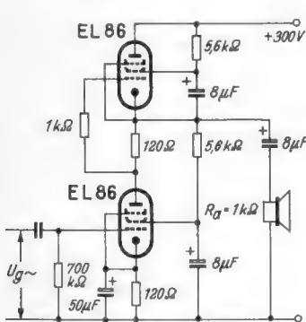
Bild 1. Einfache Schaltung einer transformatorlosen Endstufe mit zwei Röhren EL 86
