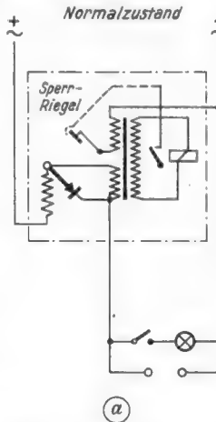
Bild 2a. Die in Bild 1a und 1b gezeigte automatische Sicherungsvorrichtung, diesmal für Wechselstromanschlus
