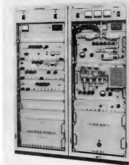
Bild 4. Modulations- und Sendergestell der Lorenz-Richtfunkanlage FM 60/120-2000
