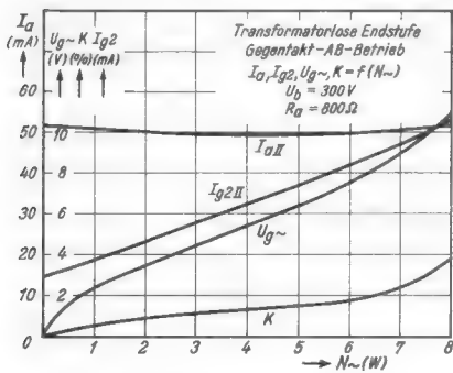
Bild 4. Stromverbrauch, Klirrfaktor und Eingangsspannungsbedarf für die Schaltung Bild 2
