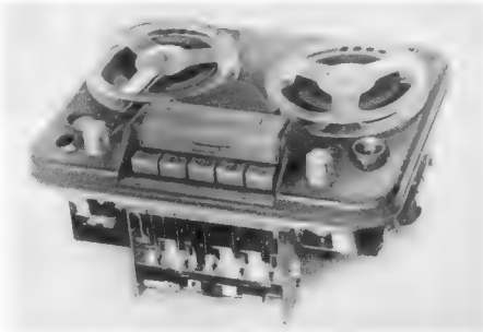
Bild 2. Ferrodyn-Junior, ein neues Bandgerät für eine Bandgeschwindigkeit von 9,5 cm/sec (AWB)
