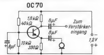
Bild 9. Mikrofon-Vorverstärker für ein Tauchpulsmikrofon mit einem Valvo-Transistor OC 70
