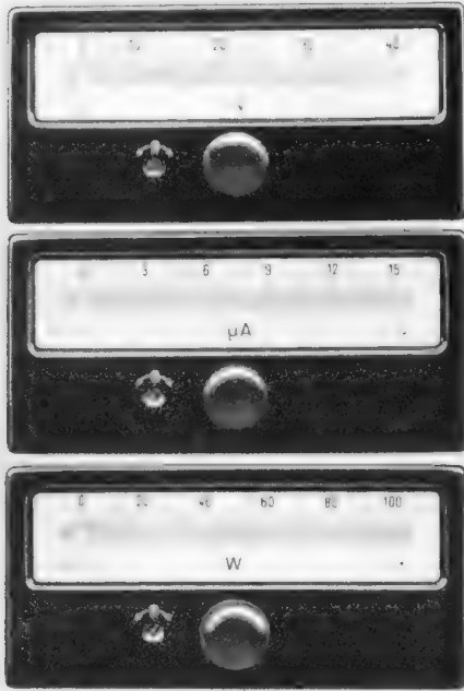
Bild 8. Drei übereinander angeordnete Betriebsinstrumente mit Lichtmarkenanzeige für Prüfplätze von Siemens & Halske
