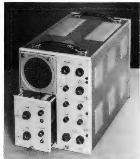
Bild 3. Zweistrahloszillograf Oscillar II von Siemens & Halske mit auswechselbarem Y-Verstärker
