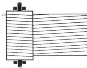
Bild 1 Druckwalze für Magnettonbänder mit gedruckten Spuren, schematisch dargestellt
