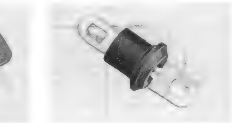
Bild 7. Ferrit-Durchführung als UKW-Drossel (Steafit-Magnesia)
