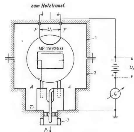
Bild 5. Prinzip des Turbatorsystems, wie es von Brown, Boveri & Cie. entwickelt wurde. FF = Heizzuführung, AA = Parallelsystem, Tr = Symmetrie/Unsymmetrie-Transformator, Po = Ausgangsleistung. 1 = zylindrisches Schutzgehäuse der Röhre, 2 = Transformatorgehäuse, 3 = Hf-Ausgangsstecker für Koaxial-Kabel
