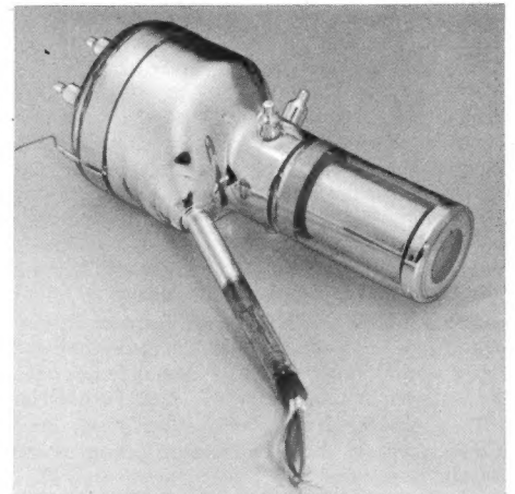
Bild 2. Die neue Fernseh-Bildaufnahmeröhre Szenioskop, die äußerlich dem Zwischenbild-Ikonoskop entspricht
