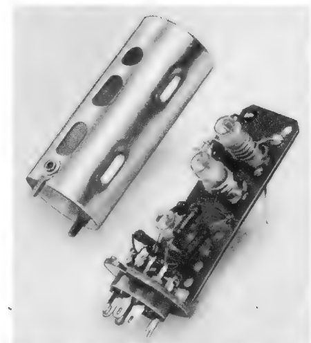
Bild 6. Bifilares T-Bandfilter mit abgenommener Abschirmung
