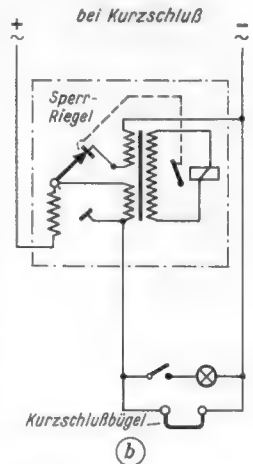
Bild 2b. Die Vorrichtung für Wechselstromanschlus bei Kurzschluß
