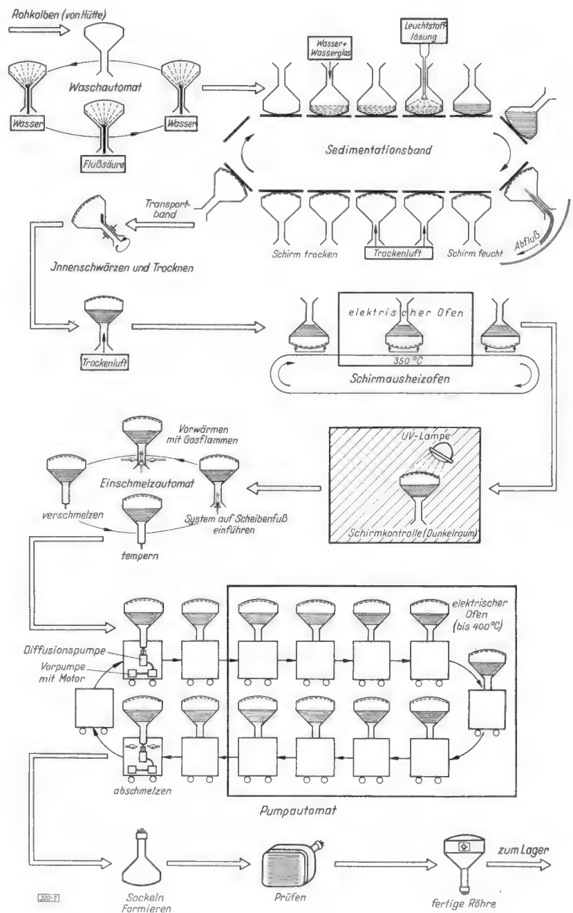
Bild 1. Schema der Bildröhrenherstellung
