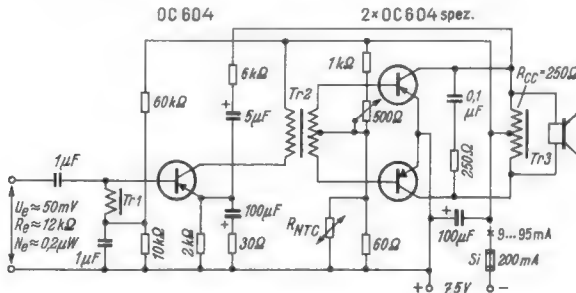
Bild 6. 0,4-W-Verstärker mit OC 604
