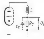
Bild 4. Zur Berechnung der Serienresonanzschaltung
