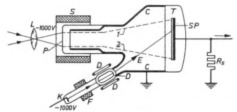
Bild 1. Schema des Zwischenbild-Ikonoskops (gilt grundsätzlich auch für das Szenioskop). L Linse, P Fotokatode, S Spule der magnetischen Elektronenlinse, T Speicherplatte, C Kollektor, E Elektronenabtastrahl, K Katode der Elektronenstrahlzeugung, F Fokussierungsspule, D Ablenkspule, SP Signalplatte, R_s Signalwiderstand
