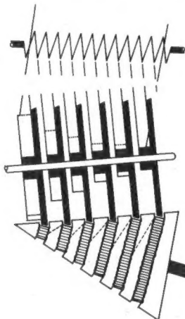
Links: Bild 2. Die oben angezeichneten Messer trennen die bedruckte Bahn in 6 mm breite Bänder, die von verschiedenen schnell angetriebenen Spulen aufgewickelt werden
