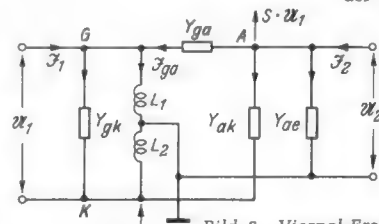
Bild 6. Vierpol-Ersatzschema der Zwischenbasisschaltung
