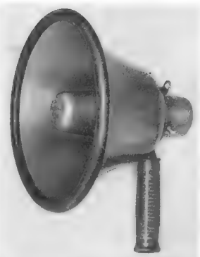
Bild 4. Isophon - Druckkammer-Handlautsprecher
