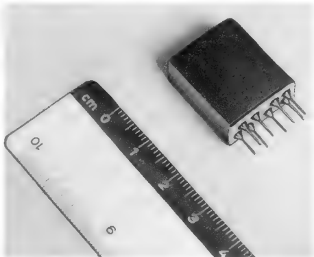
Bild 5. Das neue hermetisch abgeschlossene Mini-pol-Relais von Siemens & Halske
