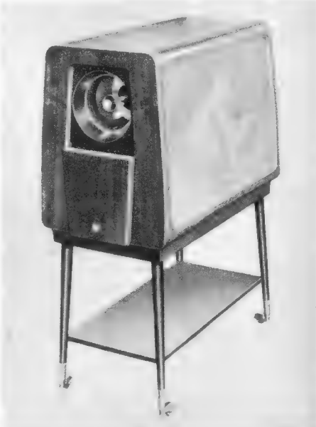
Bild 4. Grundig-Fernseh-Projektionsgerät
