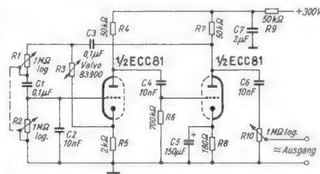
Schaltbild eines erprobten, einfachen RC-Generators für Tonfrequenzen
