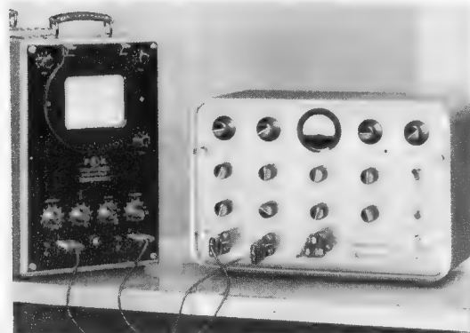
Bild 1. Meßplatz zum Aufnehmen der Kennlinienfelder von Transistoren (Vertrieb Gossen)
