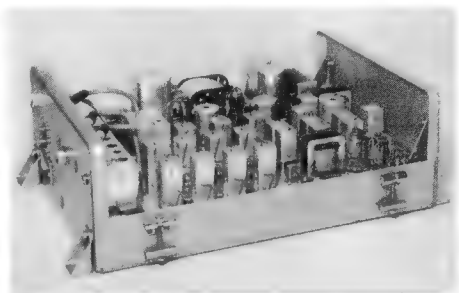
Bild 6. Fahrzeug-Funksprechanlage mit Subminiatur-Röhren (Tekade B 70)
