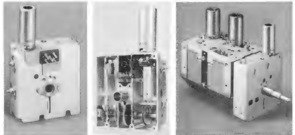
Bild 1. Der Dezi-Abstimmteil Typ 107 der Firma NSF: links Außenansicht, Mitte Innenansicht bei abgenommener Deckplatte, rechts an einen normalen Tuner angebaut
