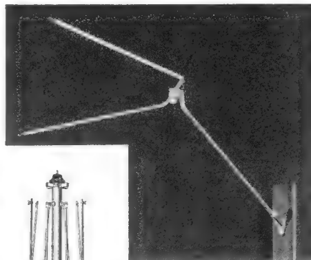
Das kleine V, ein Fernseh-Fenster-Dipol von Roka
