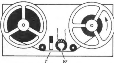
Unten: Bild 3. Anordnung des Permanentmagneten I und des Wiedergabekopfes W im Tonbandgerät. Die Remanenz braucht vom Magneten bis zum Wiedergabekopf nur \frac{1}{4} Sekunde zu halten
