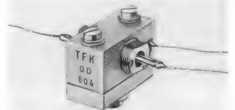
Bild 4. Ansicht des Telefunken-Leistungstransistors OD 604
