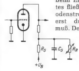
Bild 1. VDR-Widerstand parallel zum Siebkondensator einer Verstärkerröhre
