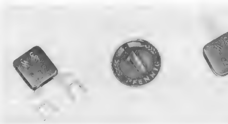
Bild 3. Zwei kunststoffumpreßte Ausführungen des Siemens-Gehörschutzgleichrichters für Kopfhörer
